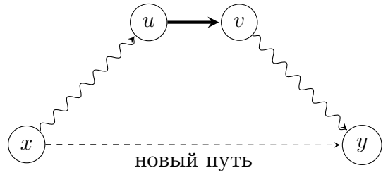
Рис. 10: Нахождение нового пути
