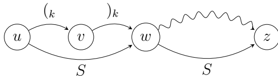
Рис. 12: Случай с меткой (k
